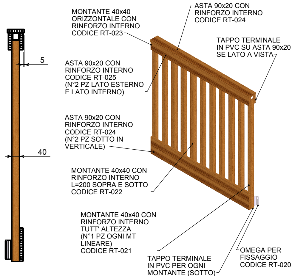
SEZIONE C-C
